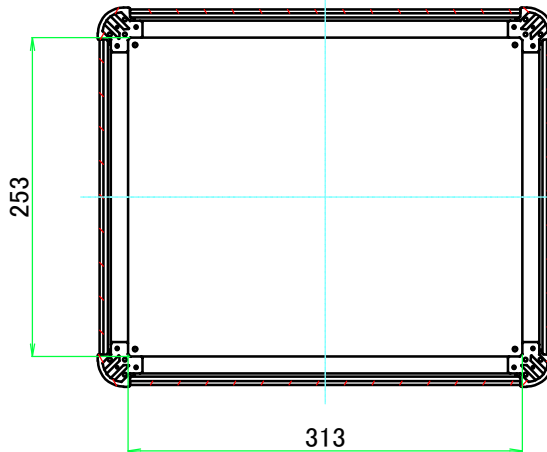
C-C ( 1 : 6 )
